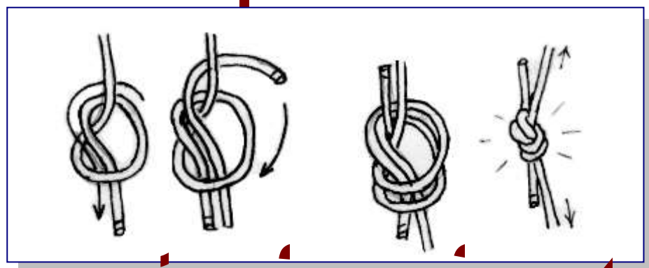
2. Hevedercsomó hevederből és kötélből kötve
